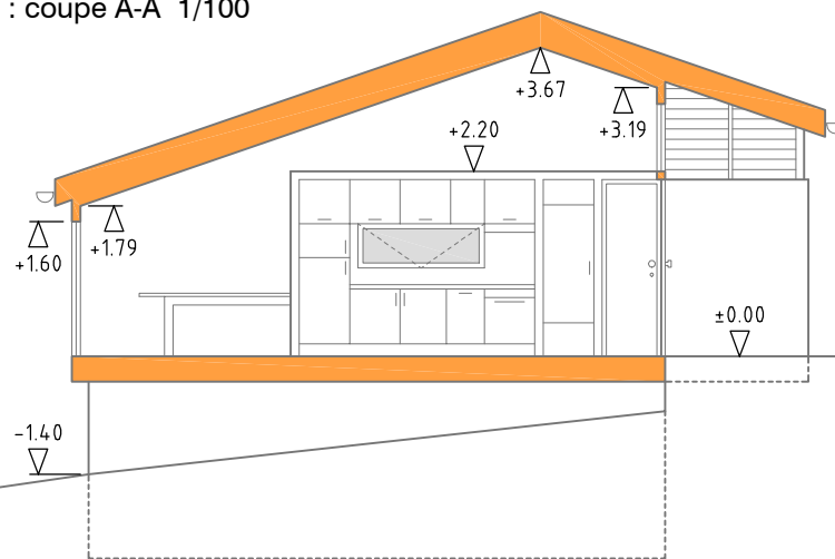
projet : coupe A-A 1/100
