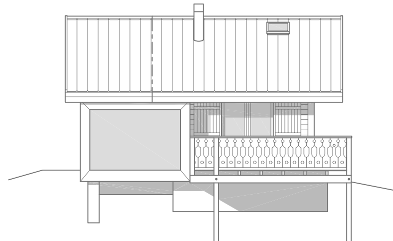
projet : facade nord 1/100
